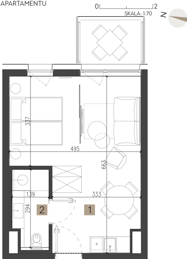
RZUT APARTAMENTU
