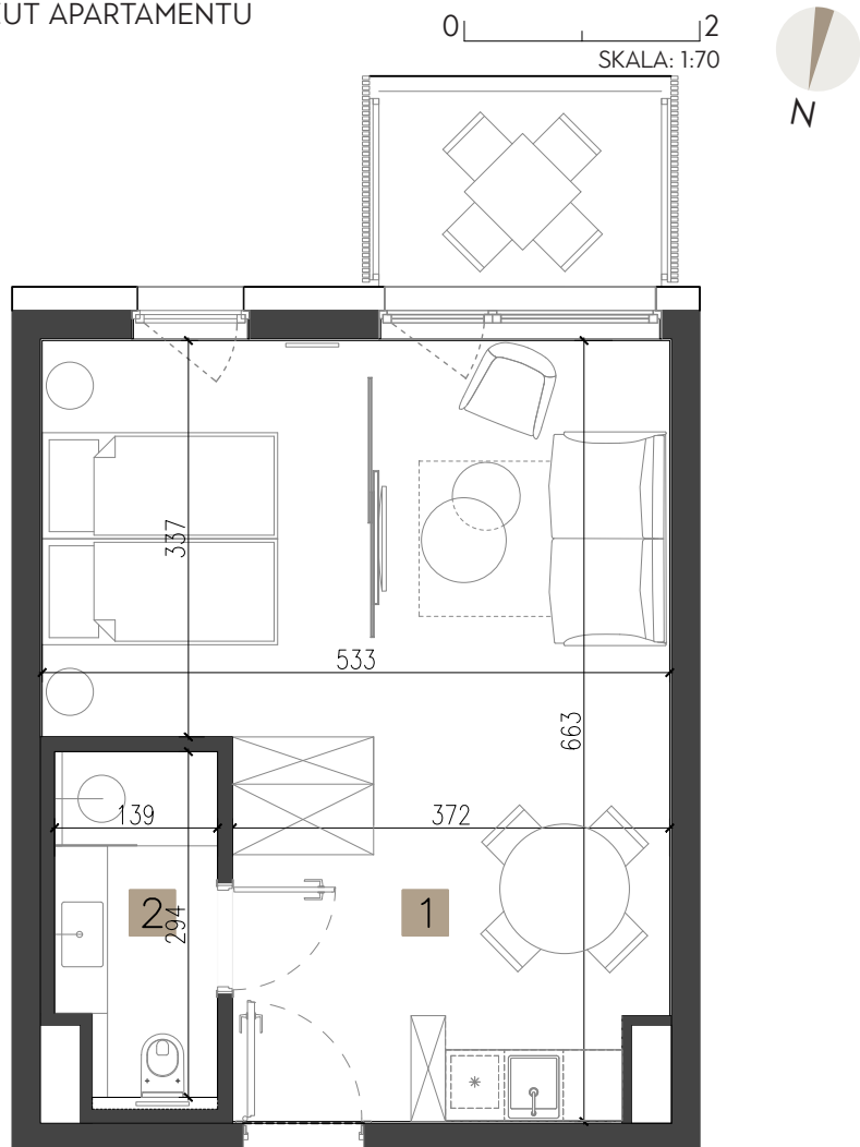
RZUT APARTAMENTU
