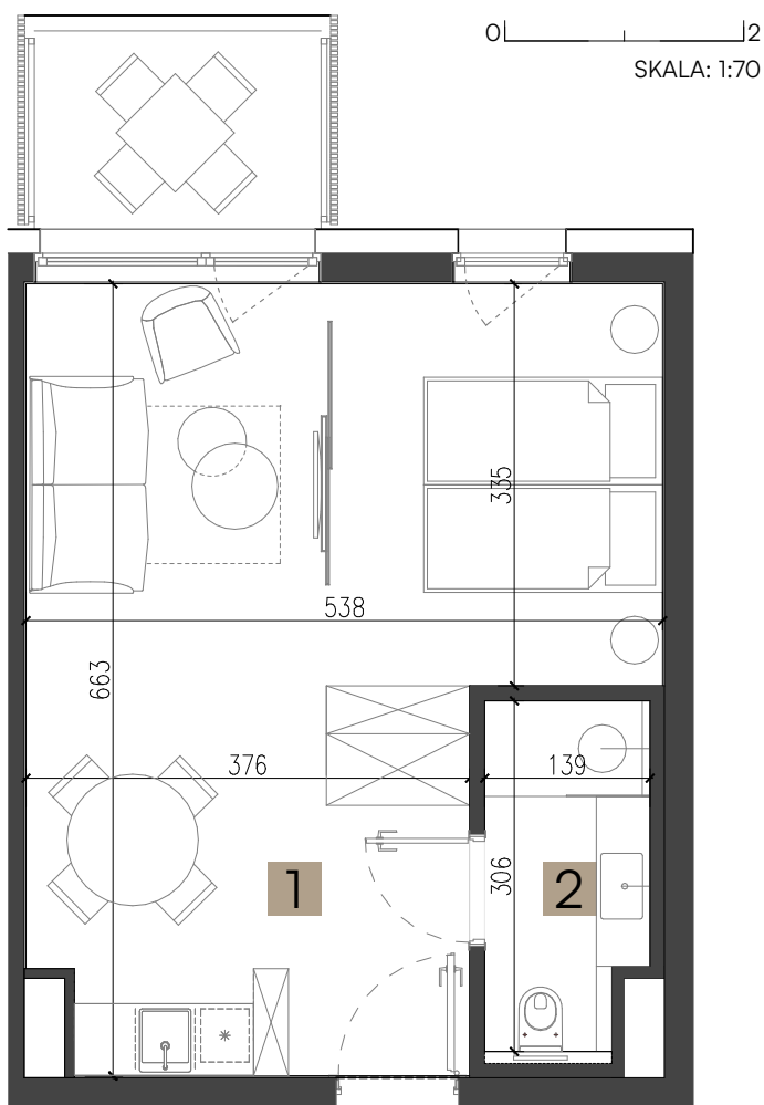
RZUT APARTAMENTU
